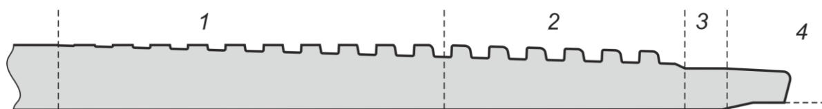
а) – Поверхность резьбового соединения ниппеля
