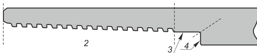
б) – Поверхность резьбового соединения муфты
