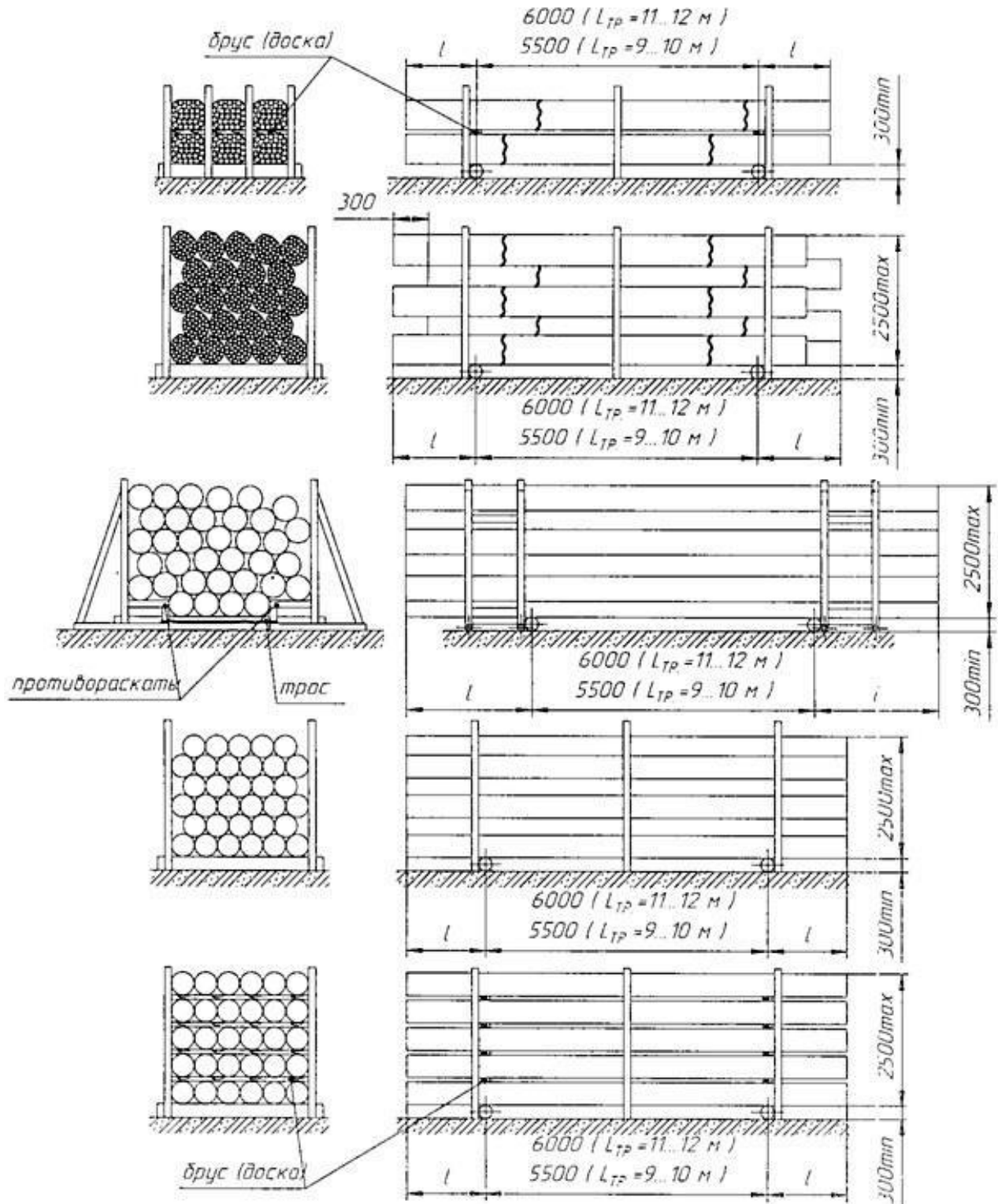
Рисунок 5 - Схемы укладки бурильных труб
