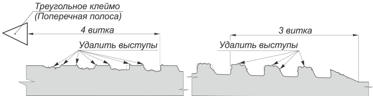
а) – Поверхность резьбового соединения ниппеля
