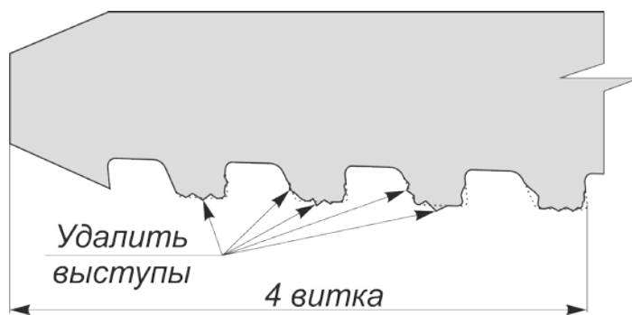
б) – Поверхность резьбового соединения муфты
